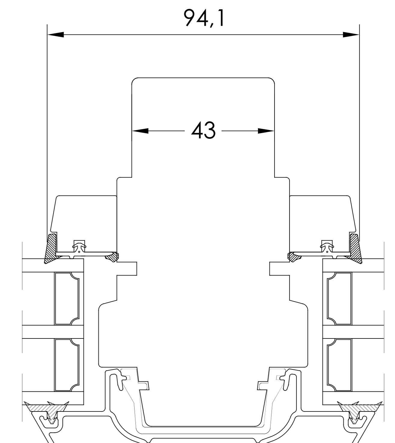
HORISONTALT SNITT TILLVAL - Flerluft Fasta delar med karmdelande post
