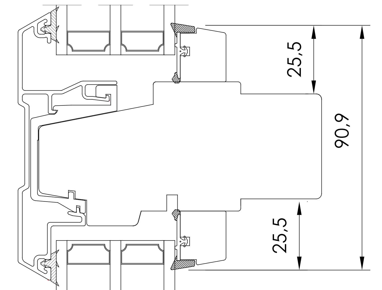
VERTIKALT SNITT TILLVAL - Flerluft Fasta delar med karmdelande tvärpost
